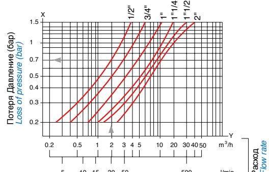
Диаграмма падения давления DROP LOSS DIAGRAM раздел B - Chart B
