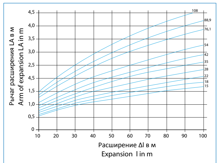
Рис. 2 – Компенсация общего расширения- Compensation of joint expansion
